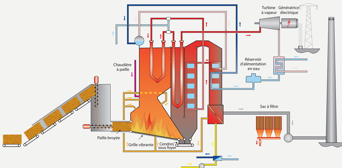
FIGURE 7 Schéma d'une turbine à vapeur alimentée par une chaudière à gradin permettant la production d'électricité à Funen, DK.
